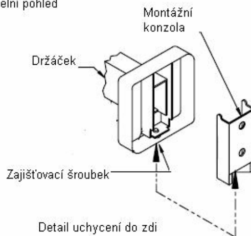
Čelní pohled
