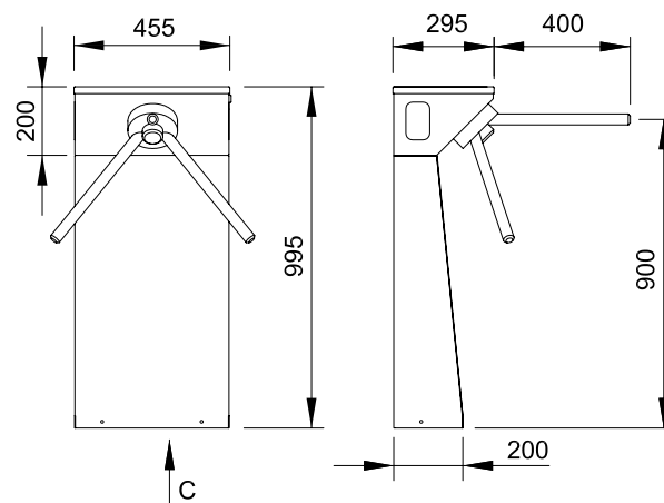
Turniket TRM 01 se stojanem STR 01
